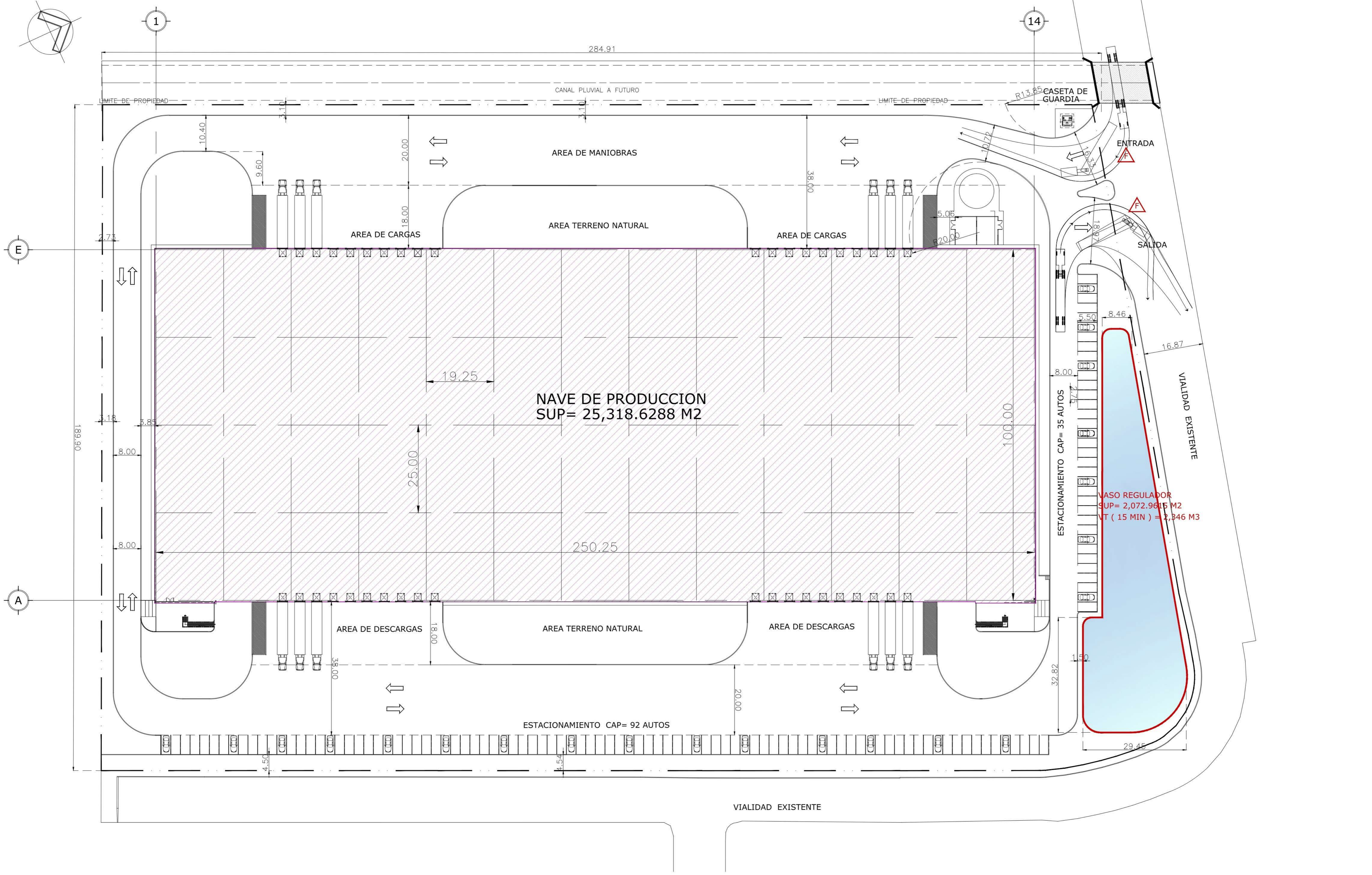
01 PLANO DE CONJUNTO OPCION CROSS DOCK ESCALA 1:500
